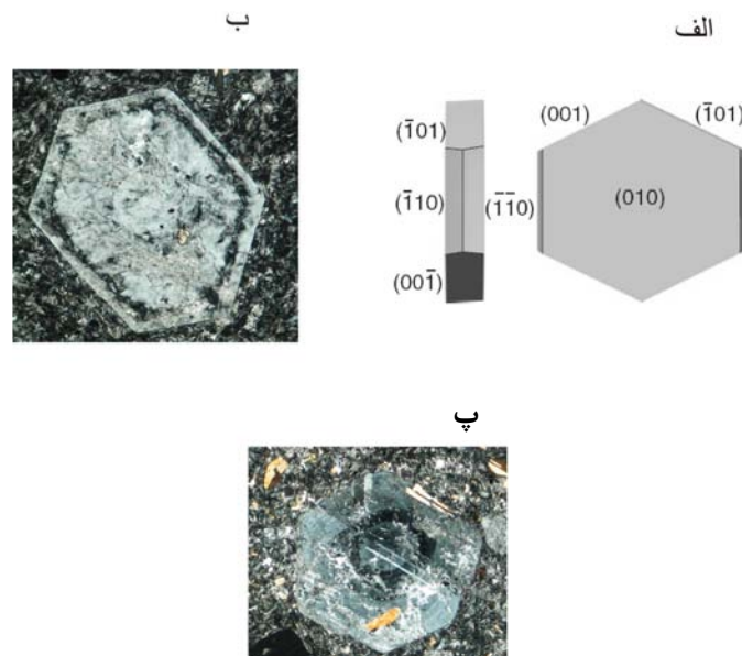
شکل ۶ الف) مدلی از یک تخته‌ی پلاژیوکلاز به‌عنوان شکل ایده‌ال یک بلور پلاژیوکلاز که با برنامه‌ی نرم‌افزاری ایجاد شده است (برگرفته از [۲۰]). در این مدل، سرعت رشد (۰۱۰) معادل با ۰٫۲ برابر سرعت رشد وجوه دیگر است. ب) بلور پلاژیوکلاز که وجه (۰۱۰) را نشان می‌دهد (مقطع KHA6). پ) وجه تخته‌ای بلور پلاژیوکلاز در مقطع KHD2 به موازات (۰۱۰) آن دیده می‌شود.
