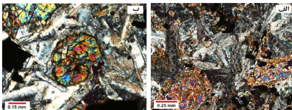
شکل ۴ درشت بلورهای کلینوپیروکسن‌های تمام شکل‌دار و نیمه شکل‌دار در دولریت‌های منطقه.
