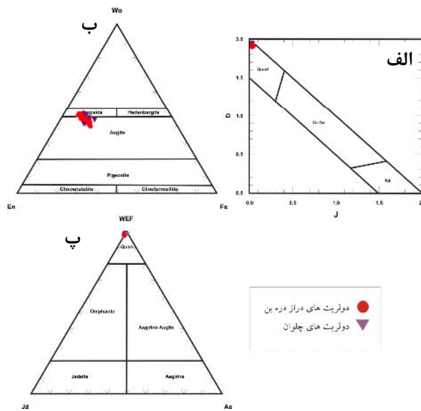
شکل ۷ نتایج تجزیه‌ی نقطه‌ای کلینوپیکروکسن‌های سنگ‌های نیمه عمیق منطقه [۱۱]. الف) نمودار کوارتز - ژادئیت (ب) نمودار هس (پ) بروی نمودار کوارتز - ژادئیت - آکمیت .
