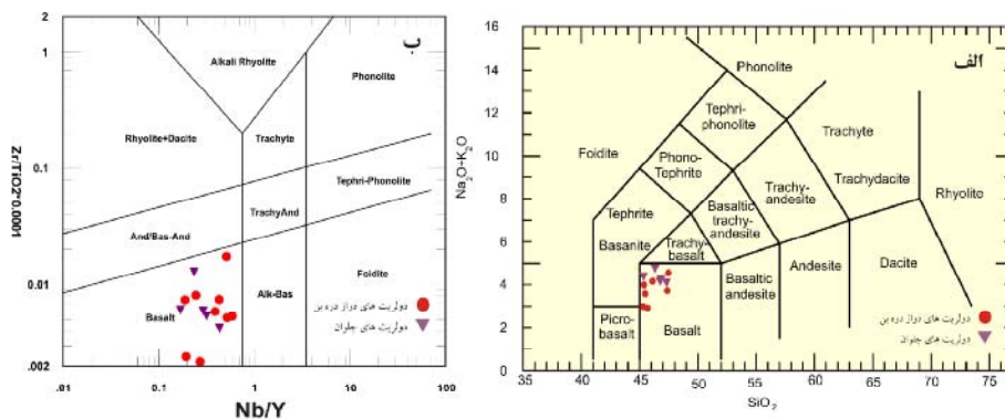
شکل ۲ رده بندی ژئوشیمیایی و نام گذاری سنگ های منطقه مورد بررسی.
