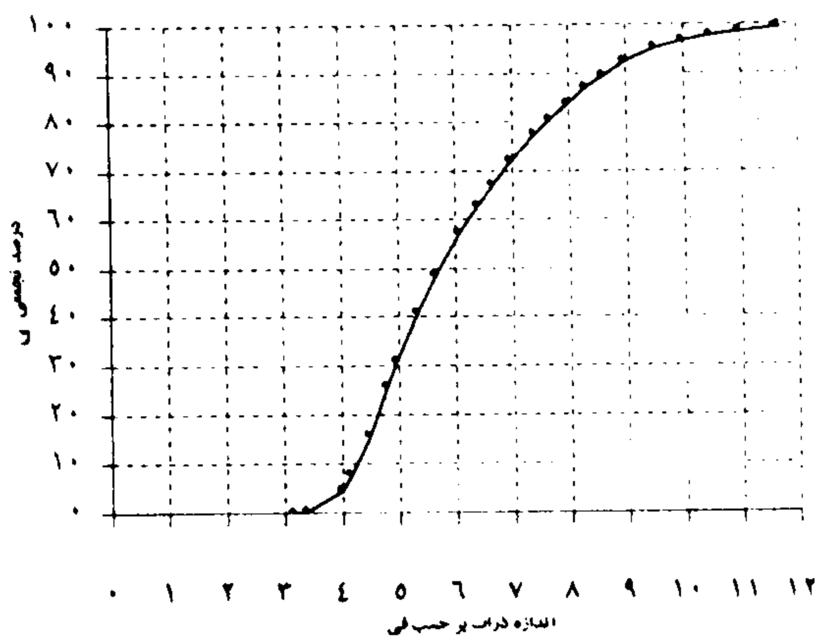
شکل (۴) منحنی تجمعی اندازه ذرات نمونه (Loess-2)
