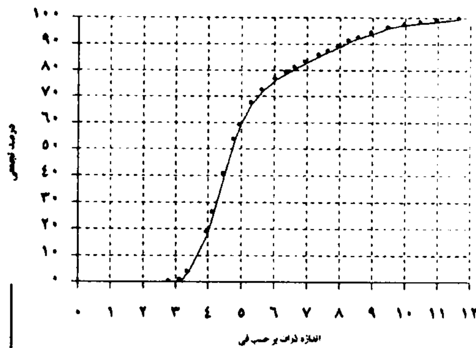
شکل (۹) منحنی تجمعی اندازه ذرات نمونه (Loess-6)
