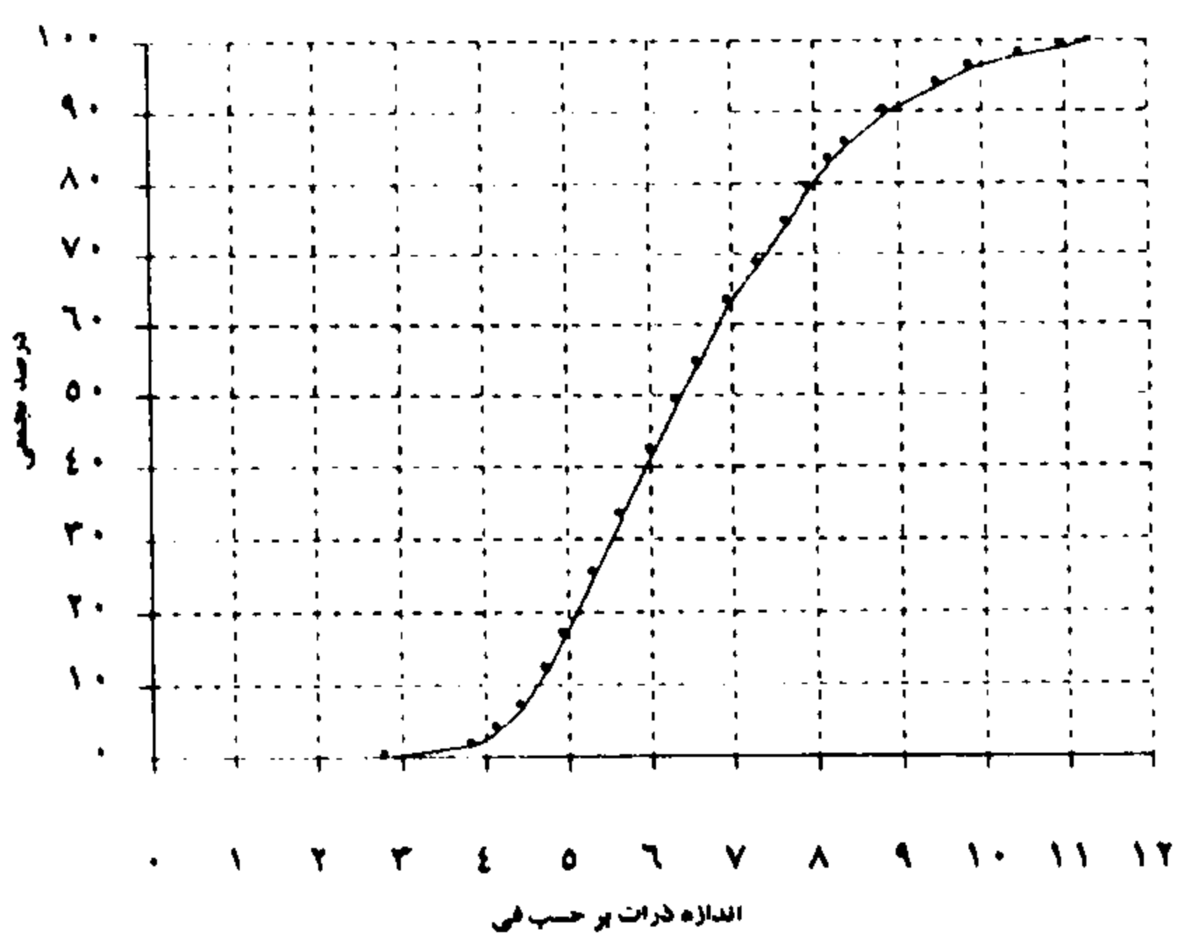
شکل (۷) منحنی تجمعی اندازه ذرات نمونه (Loess-3)
