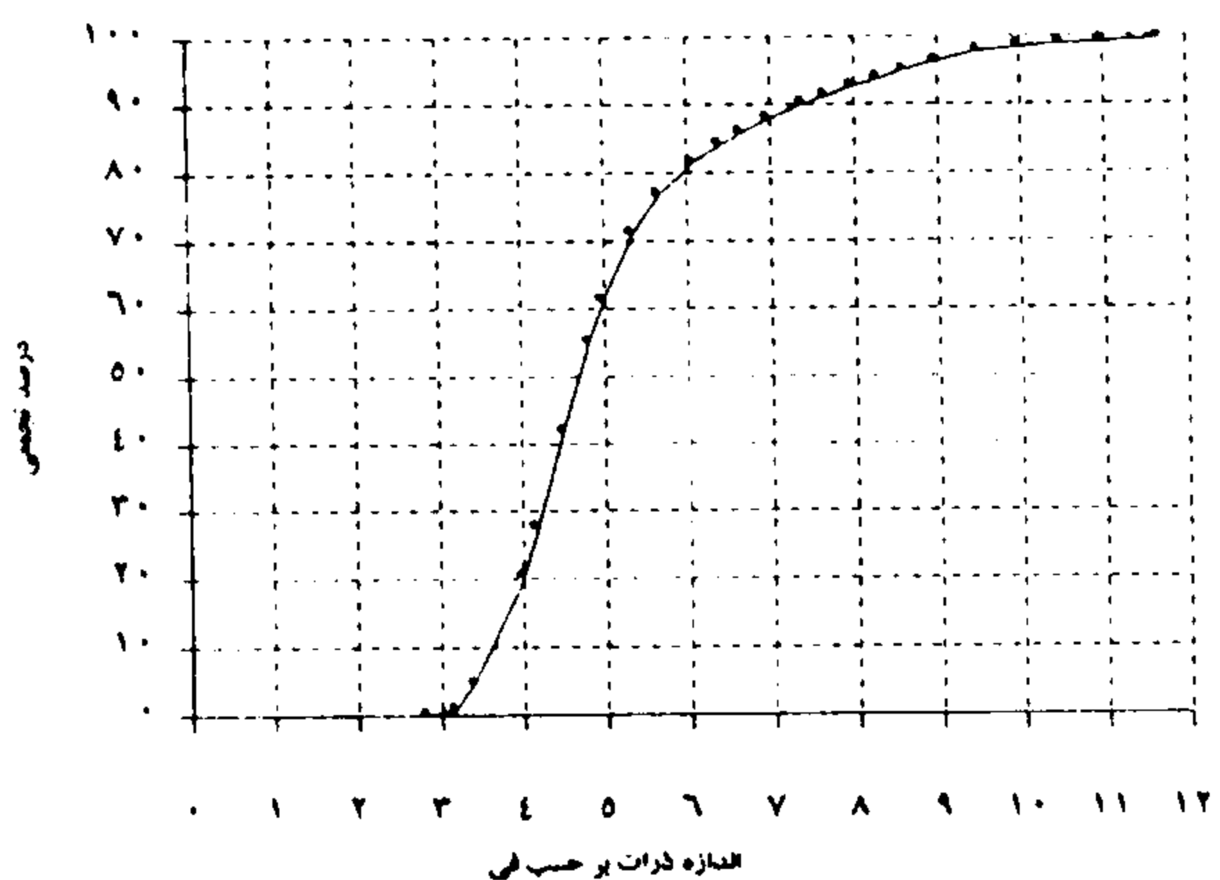
شکل (۵) منحنی تجمعی اندازه ذرات نمونه (Loess-1)
