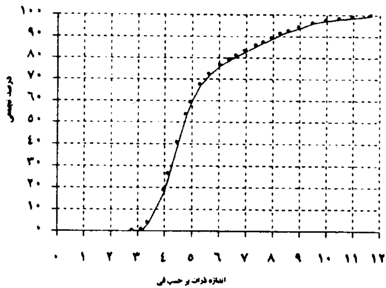
شکل (۸) منحنی تجمعی اندازه ذرات نمونه (Loess-5)
