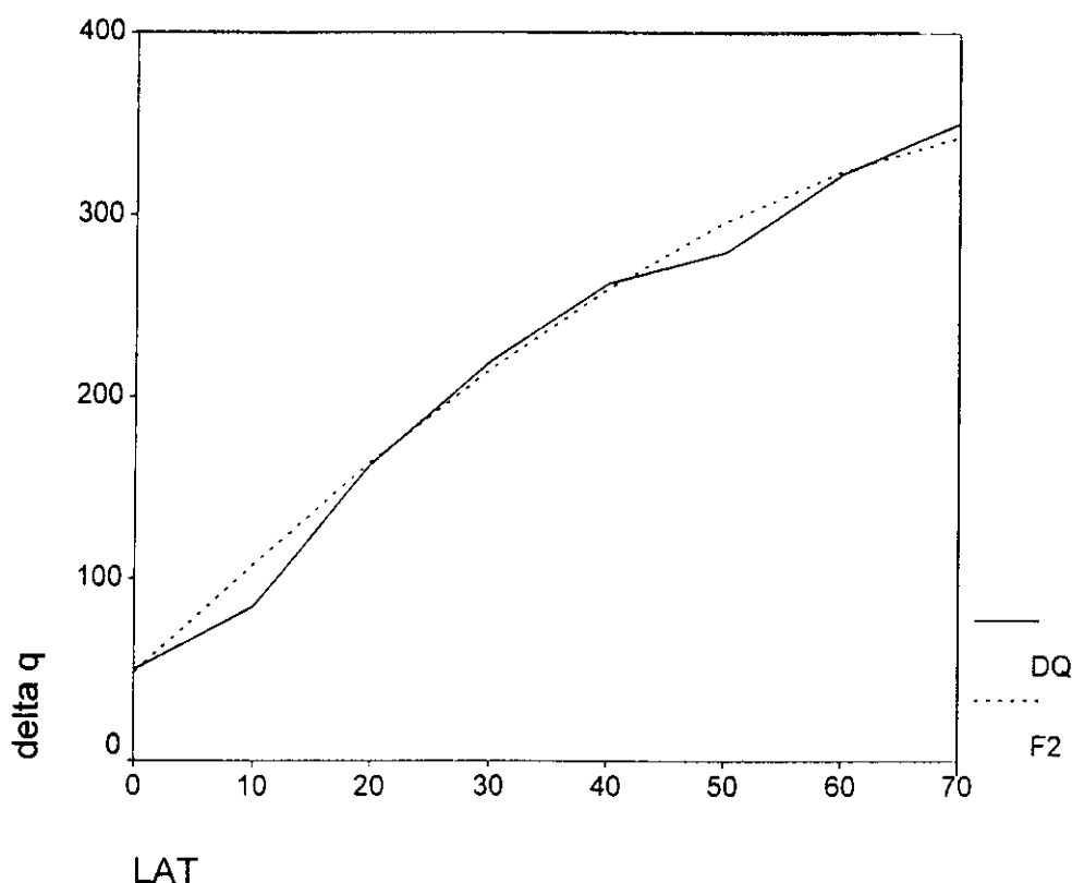
شکل ۱- برازش دامنه نوسان، موازنه تابش، موازنه مشاهده شده (DQ) و دامنه نوسان موازنه تابش برآورد شده (F2) براساس 350\sin(\varphi+8^\circ) در عرض‌های جغرافیایی مختلف
