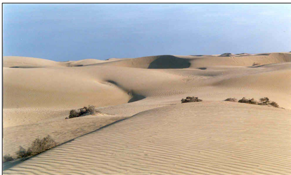
شکل ۲- تپه‌های ماسه‌ای مرگب در منطقه ساحلی درک.
