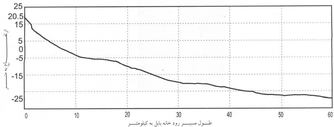
شکل ۳ - نیمرخ طولی رودخانه بابل در محدوده جلگه ساحلی
