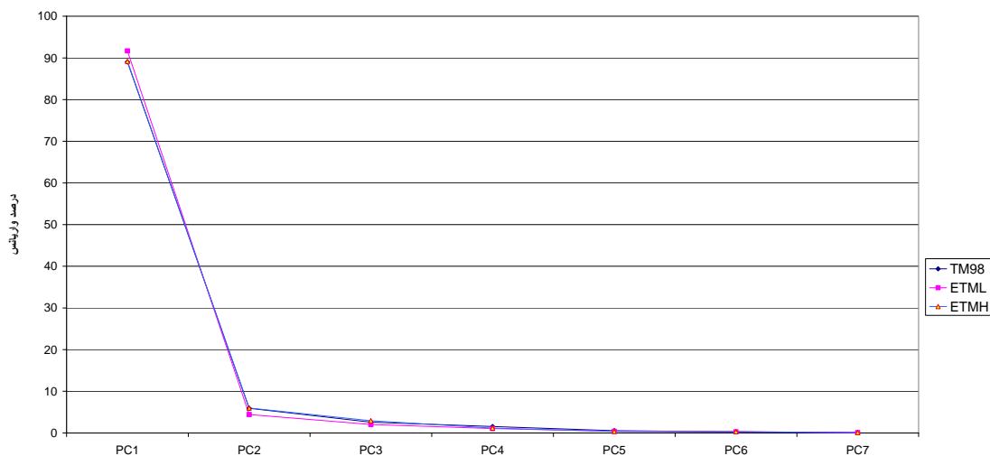
شکل ۱۶- مقایسه درصد واریانس در مؤلفه های مختلف PCA در سنجنده های TM و ETM+
