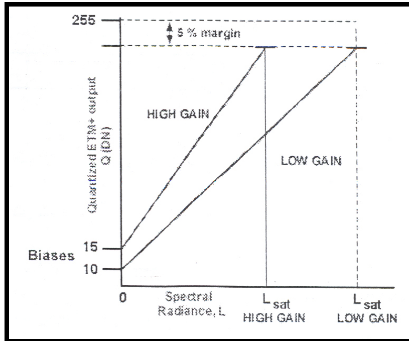
شکل ۱- محدوده Low Gain و High Gain در تصاویر سنجنده ETM+
