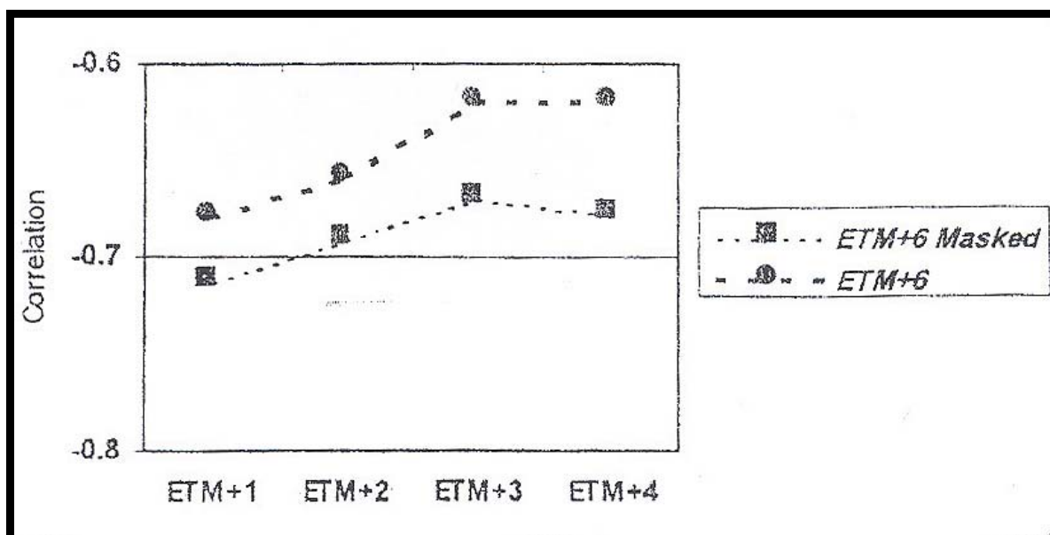
شکل ۱۱- نمودار روند همبستگی بین باند ترمال و باندهای انعکاسی در سنجنده ETM+
