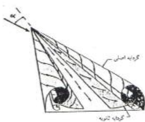
شکل ۲- گردابه‌های اصلی و ثانویه روی بال
