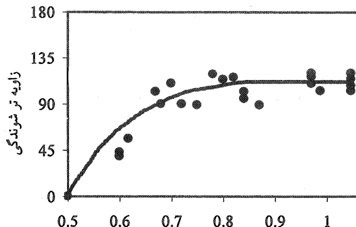
شکل ۱- زاویه تر شوندهگی کاربرد تیتانیوم توسط مس مذاب برحسب تایی از نسبت C/Ti [%].
