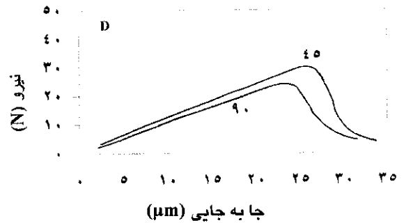
شکل ۸- منحنی نیرو- جا به جایی برای نمونه D در 1000^{\circ}\text{C} برای دو زمان نگهداری ۹۰ و ۴۵ دقیقه
