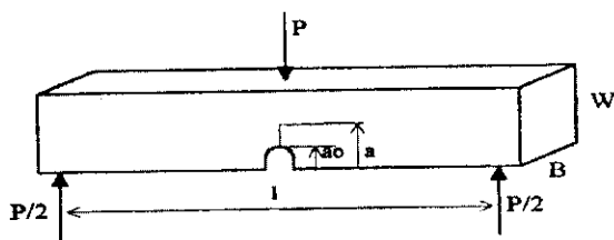
شکل ۳- نمایش شماتیکی آزمایش خمش سه نقطه‌ای در جهت رسم منحنیهای R
