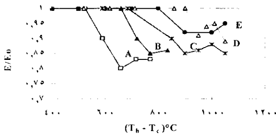
شکل ۱۱- تغییرات نسبی مدول یانگ بر حسب \Delta T اعمال شده
