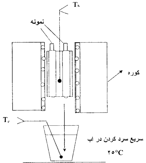
شکل ۵- نمایش شماتیکی عملیات شوک گرمایی با غوطه‌وری در آب
