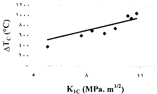
شکل ۱۲- مقادیر \Delta T_c در برابر K_{IC} برای نمونه‌های مختلف
