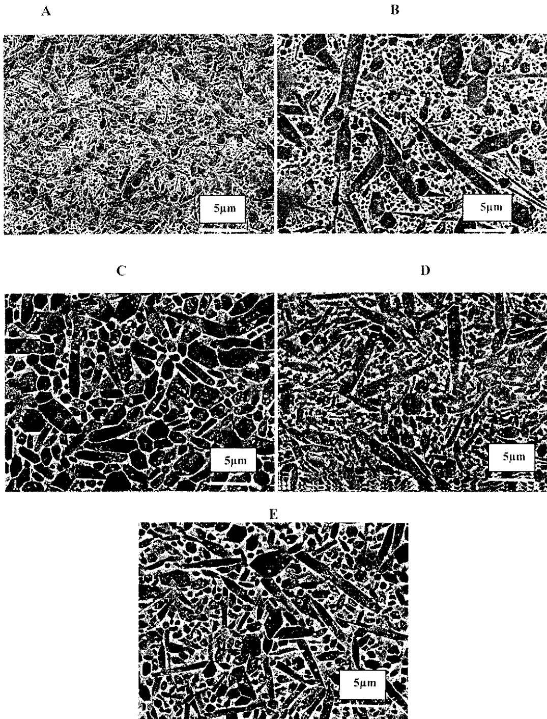
شکل ۲- تصاویر میکروسکوپ الکترونی برای پنج نمونه نیتروسلیسیم تهیه شده در شرایط مختلف
