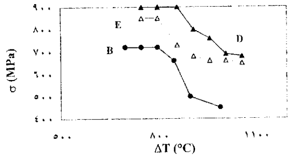
شکل ۱۴- تغییرات استحکام شکست نمونه‌های B ، D ، E و نسبت به \Delta T برای سیکل‌های شوک گرمایی مختلف
