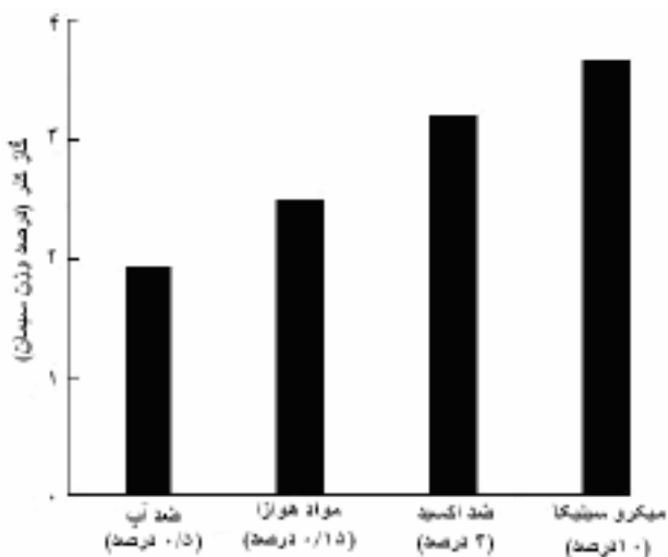
شکل ۱۰- تاثیر افزودنیها بر مقدار نفوذ کلر
