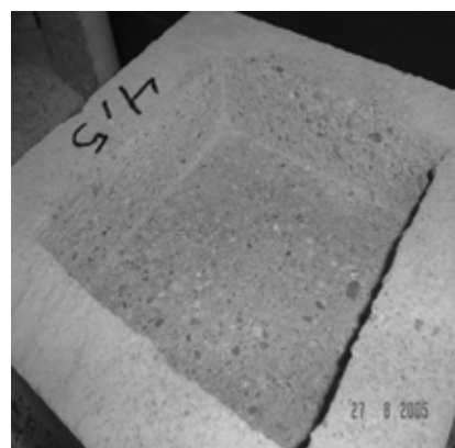
شکل ۳- نمونه آزمایش کشش مستقیم
