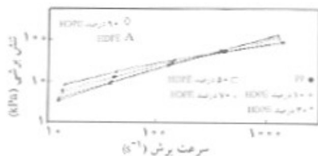
شکل ۴- تغییرات تنش برشی بر حسب سرعت برش آمیزه B1 در دمای ۲۳°C.
