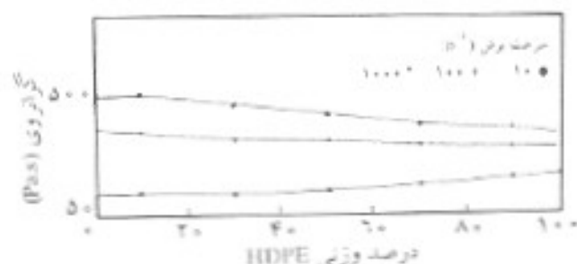
شکل ۷- تغییرات گرانروی - غلظت آمیزه B1 در دمای ۲۳°C.
