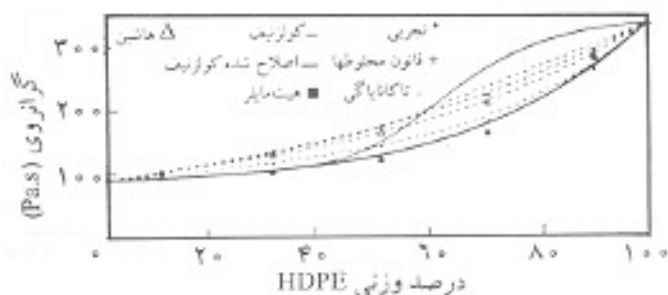
شکل ۱۲ - مقایسه نتایج آزمایشهای آمیزه B۳ با نتایج پیشینی شده از چند مدل تجربی در دمای 23^{\circ}\text{C} و سرعت برش 1000\text{ s}^{-1} .
