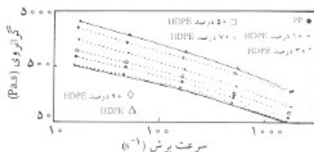
شکل ۲- تغییرات گرانروی بر حسب سرعت برش آمیزه B2 در دمای 230^\circ\text{C} .
