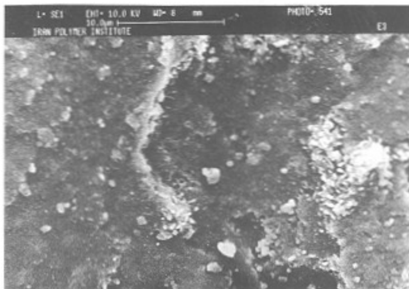
شکل ۹- سطح شکست آلیاژ PVC/ABS/NBR: ۶۰/۴۰/۳۰ یکبار اکستروود شده با بزرگنمایی ۳۰۰۰.
