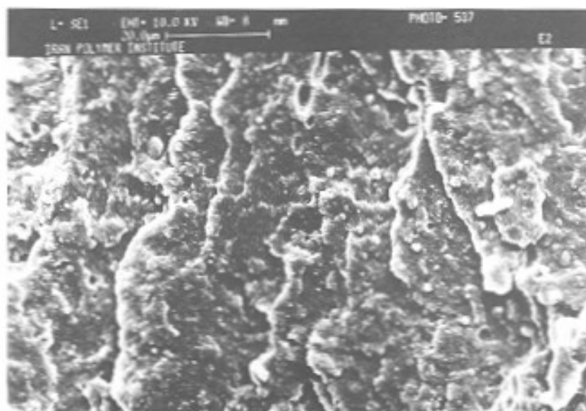
شکل ۷- سطح شکست آلیاز ۶۰/۴۰/۲۰ PVC/ABS/NBR یکبار اکستروود شده با بزرگنمایی ۸۰۰۰.
