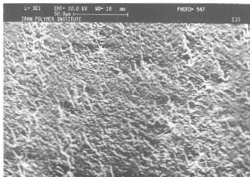
شکل ۱۰- سطح شکست آلیاژ PVC/ABS/NBR: ۶۰/۴۰/۳۰ دوبار اکستروود شده با بزرگنمایی ۵۰۰.
