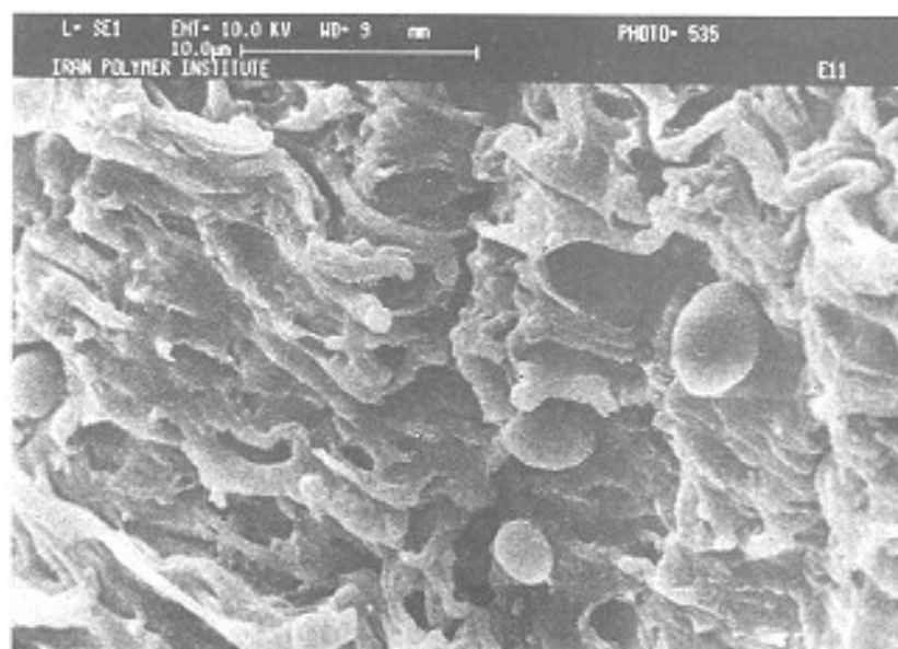
شکل ۶- سطح شکست آلیاژ ۶۰/۴۰/۱۰ PVC/ABS/NBR دوبار اکستروود شده با بزرگنمایی ۳۰۰۰.
