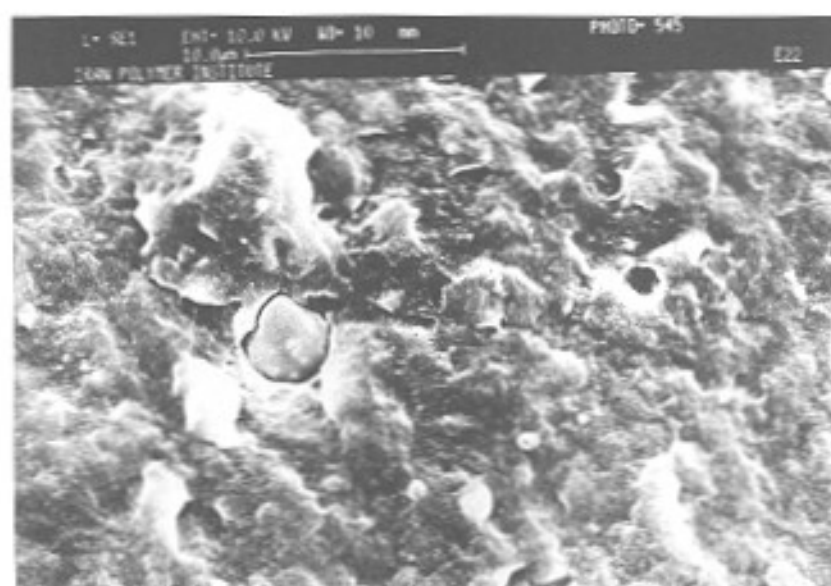
شکل ۸- سطح شکست آلیاز ۶۰/۴۰/۲۰ PVC/ABS/NBR دوبار اکستروود شده با بزرگنمایی ۳۰۰۰.
