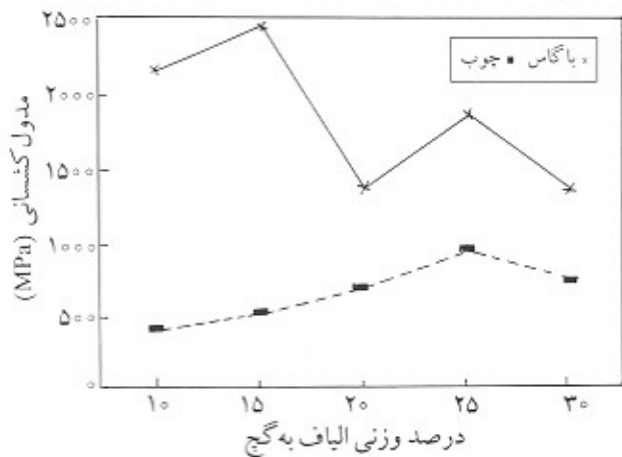
شکل ۷- تغییرات مدول کشسانی نخته‌های دارای الیاف چوب و الیاف باگاس با درصدهای وزنی متفاوت الیاف به گچ.
