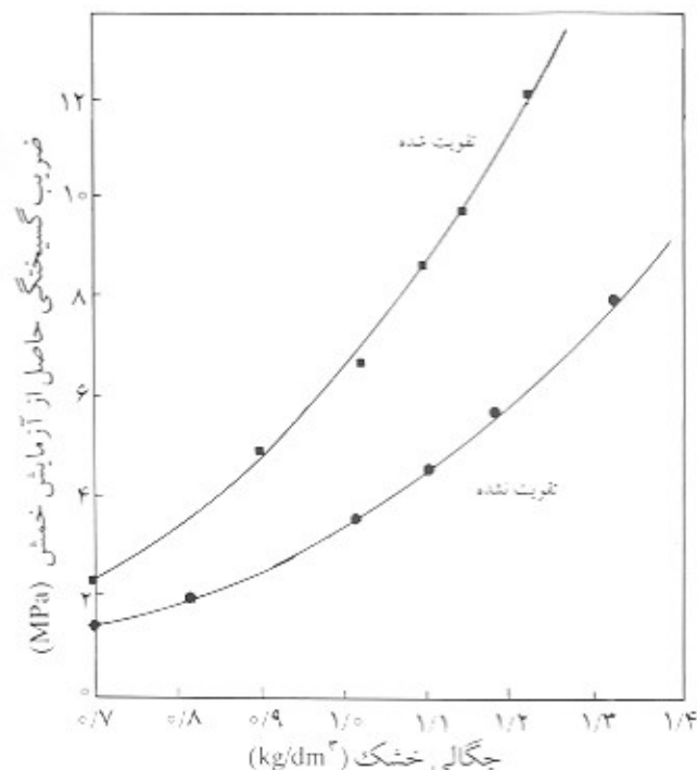
شکل ۱- ضریب گسیختگی حاصل از آزمایش خمش برای گچ تقویت شده و تقویت نشده در برابر جگالی.
