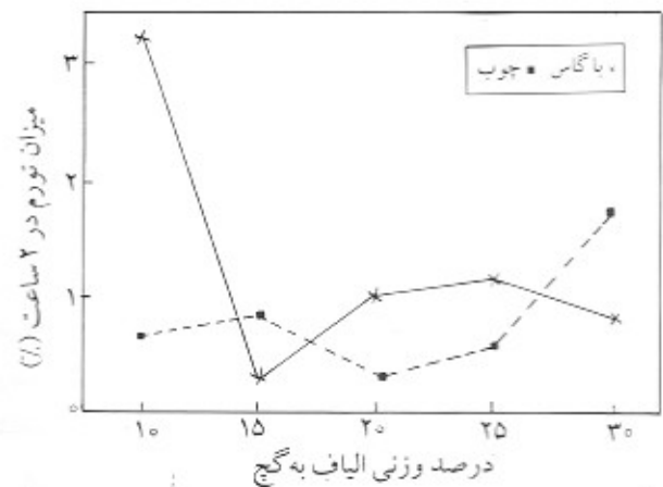
شکل ۴- تغییرات تورم پس از ۲ ساعت برای نخته‌های دارای الیاف چوب و الیاف باگاس با درصدهای وزنی متفاوت الیاف به گچ.
