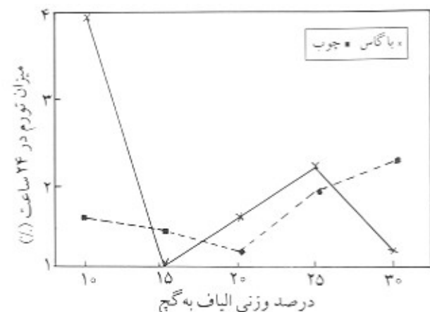
شکل ۵- تغییرات تورم پس از ۲۴ ساعت برای نخته‌های دارای الیاف چوب و الیاف باگاس با درصدهای وزنی متفاوت الیاف به گچ.
