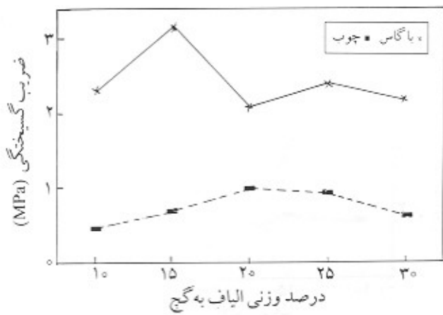
شکل ۶- تغییرات ضریب گسیختگی نخته‌های دارای الیاف چوب و الیاف باگاس با درصدهای وزنی متفاوت الیاف به گچ.
