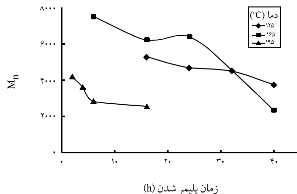
شکل ۶- اثر دما و زمان واکنش بر متوسط عددی وزن مولکولی پلی (L-لاکتید).
