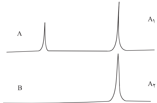
شکل ۹ - طیف ماده خالص A و B.
