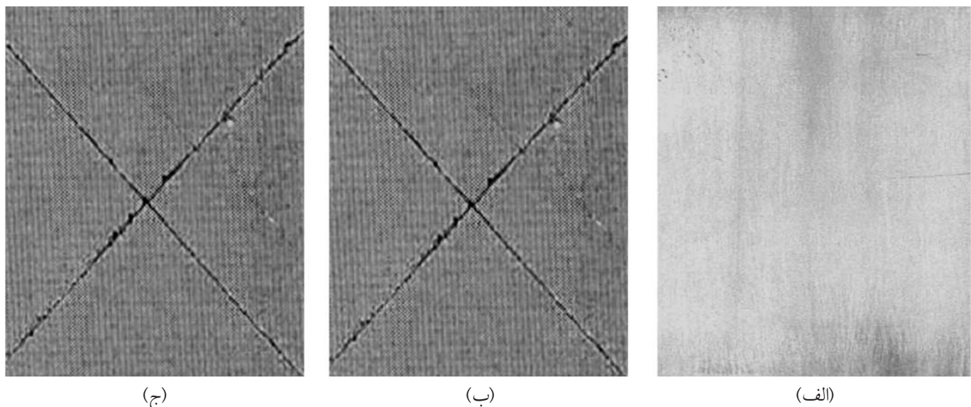
شکل ۷ (الف) سطح آلومینیم بدون پوشش هیبریدی، (ب) نمونه با پوشش هیبریدی قبل از انجام آزمون پاشش مه نمک و (ج) نمونه با پوشش هیبریدی بعد از انجام آزمون پاشش مه نمک.
