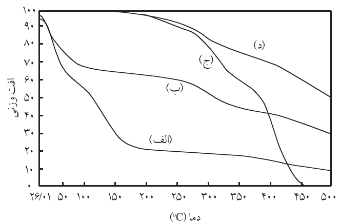
شکل ۴ دمانگاشت TGA: (الف) فاز معدنی، (ب) فاز هیبریدی آلی - معدنی قبل از پخت، (ج) فاز آلی و (د) فاز هیبریدی آلی - معدنی بعد از پخت با سرعت گرمادهی 10\text{ }^{\circ}\text{C}/\text{min} .
