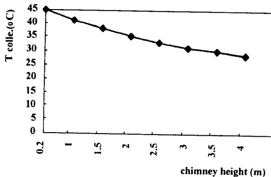
نمودار ۶: تاثیر ارتفاع دودکش بر دمای هوا در خروج از جمع کننده.
