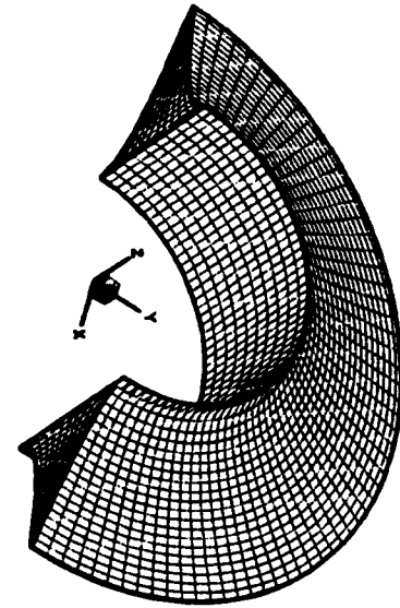
شکل ۵: شبکه پره با پروفیل سهموی.
