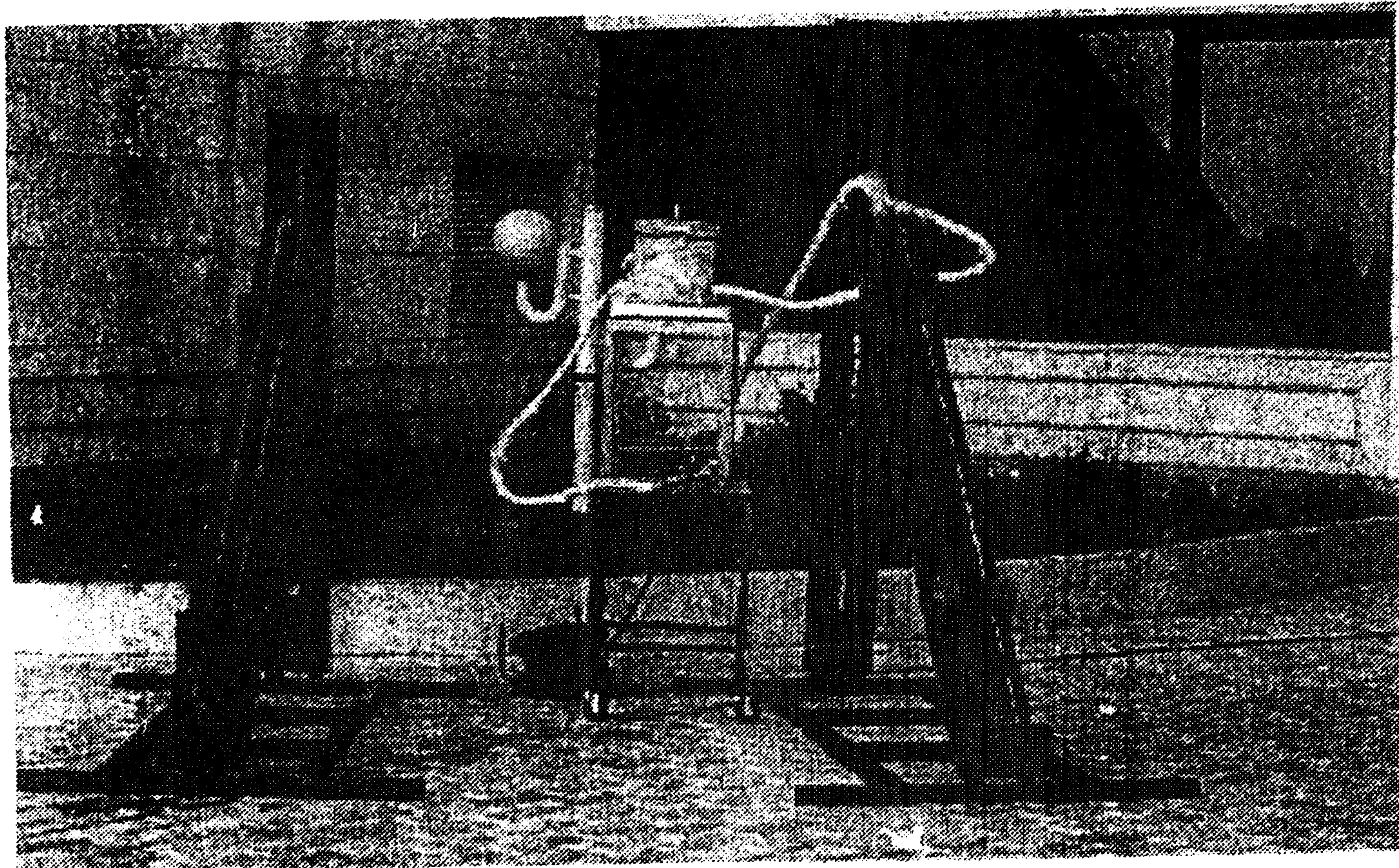
شکل ۳: نمونه ترموسیفون خورشیدی که در مرکز توسعه انرژی‌های نو ساخته و مورد آزمایش قرار گرفت.
