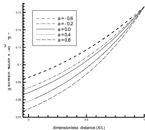
شکل ۵- اثر شتاب خطی بر شعاع موئینگی مایع
