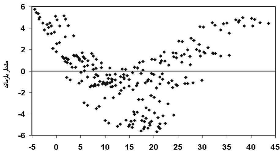
شکل ۴: نمودار مقادیر بازماند در مقابل مقادیر پراش داده شده. ANOVA مقادیر پیریت پوشش نیافته (٪) پیش‌بینی شده توسط
