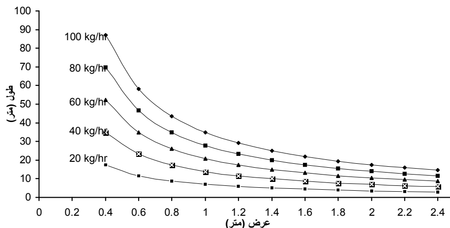
شکل ۱۸: نمودار طول خشک کن بر حسب عرض در هر مقدار از سرعت محصول خشک نهایی در شرایط عبور ۳۰٪ هوای اضافی.
