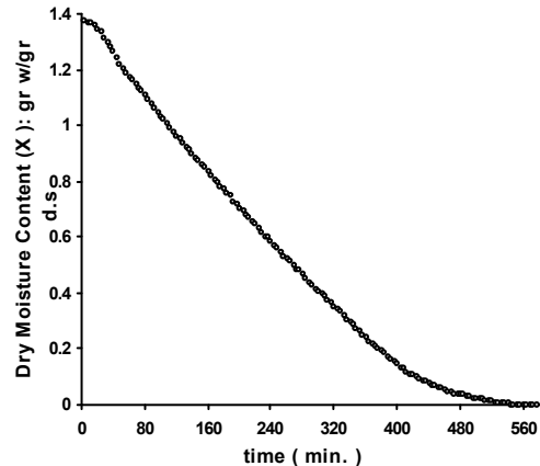
شکل ۳: منحنی خشک کردن برای آزمایش
