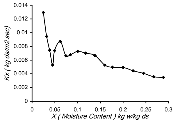
شکل ۱۷: پروفایل ضریب انتقال جرم جامد مرطوب در بخش ممانعی حاصل از آزمایشهای سینتیکی.
