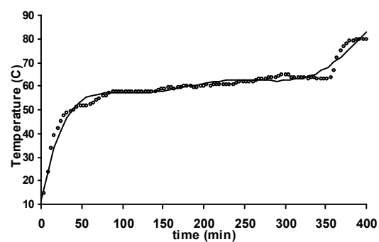
شکل ۴: منحنی دما - زمان برای آزمایش
