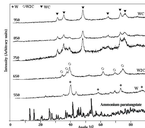
شکل ۱: طیف‌های XRD نمونه‌های حاصل از واکنش پاراتنگستات آمونیوم در مخلوط گازی ۲۰٪ متان در هیدروژن با نرخ افزایش دمای ۳۳°C/min تا دماهای نهایی مابین ۳۵۰ تا ۹۵۰°C در مقایسه با پاراتنگستات آمونیوم.
