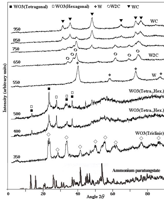
شکل ۲: طیف‌های XRD نمونه‌های حاصل از واکنش پاراتنگستات آمونیوم در مخلوط گازی ۲۰٪ متان در هیدروژن با نرخ افزایش دمای ۱°C/min تا دماهای نهایی مابین ۵۵۰ تا ۹۵۰°C در مقایسه با پاراتنگستات آمونیوم.
