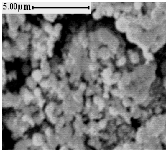
شکل ۹: تصویر SEM از نمونه حرارت داده شده تا دمای نهایی 850^\circ C تحت شیب حرارتی 5^\circ C/min بعد از سرد شدن تا دمای محیط.
