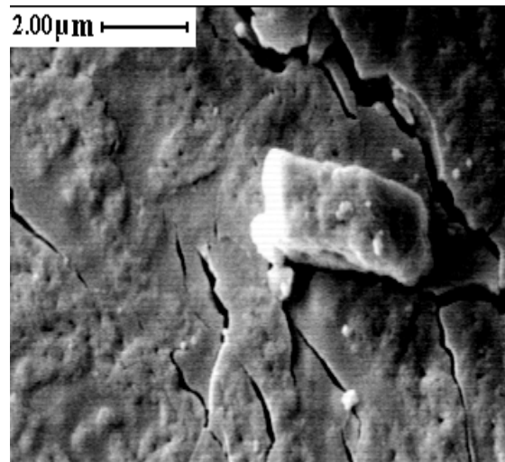
شکل ۸: تصویر SEM از نمونه حرارت داده شده تا دمای نهایی 850^\circ C تحت شیب حرارتی 1^\circ C/min بعد از سرد شدن تا دمای محیط.
