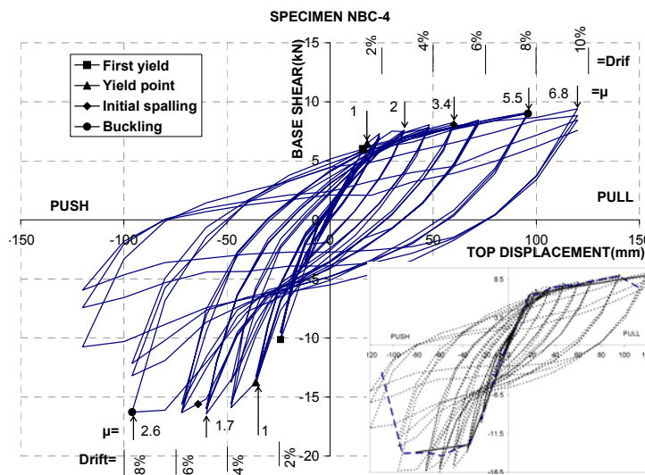
شکل ۵: نمودار دررفت-مقاومت جانبی برای نمونه نیمه مهندسی تیر طبقات زیرین، ۴ - NBC.
