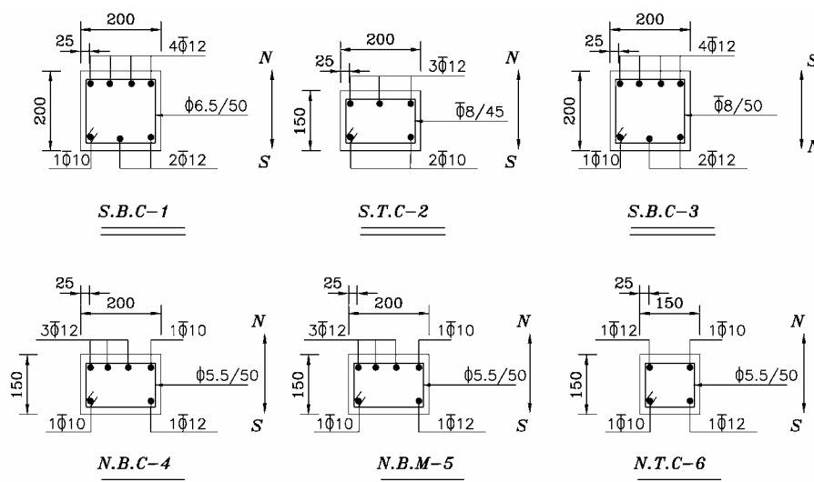
شکل ۱: جزئیات نمونه‌های آزمایشگاهی (واحد ها بر حسب mm می باشد).
