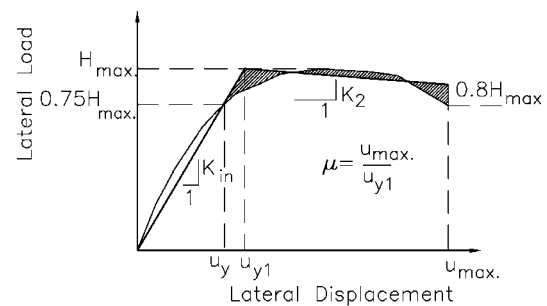
شکل ۱۱: تعریف منحنی ایده‌آل شده.
