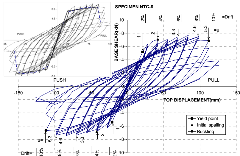
شکل ۴: نمودار تغییرشکل-مقاومت جانبی برای نمونه نیمه مهندسی تیر طبقات فوقانی، ۶ - NTX.
