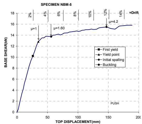
شکل ۶: نمودار مقاومت جانبی در برابر تغییر شکل از نمونه NBM - 5.
