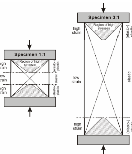
شکل ۱۲: تاثیر سطوح انتهایی در شکلهای مختلف نمونه [۸].
