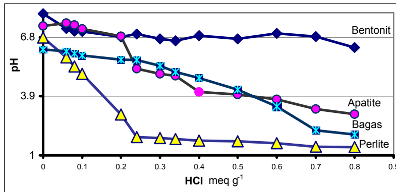
شکل ۱- نمودار تیتراسیون آپاتیت، پرلیت، بنتونیت و باگاس با HCl
