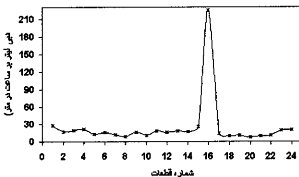
شکل ۳ - تغییرات دبی جریان در طول لوله تراوا در انتهای آزمایش (۸ ساعت) در فشار ۱۵ متر
