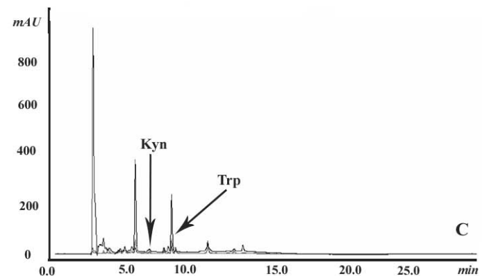
نمودار ۵- نمونه‌ای از منحنی‌های خروج کینورین و تریپتوفان از ستون C18. A- منحنی مربوط به تزریق نمونه‌های استاندارد؛ همانطور که نشان داده شده است در شرایط آزمایش کینورین تقریباً ۶/۵ دقیقه و تریپتوفان تقریباً ۸ دقیقه بعد از تزریق از ستون خارج می‌شود. میزان جذب در دو طول موج ۲۲۰nm و ۲۵۴nm اندازه‌گیری شده است. B- منحنی مربوط به تزریق مایع رویی کشت MLR سلول‌های دندریتیک تیمار شده با سرم موش غیرباردار می‌باشد. میزان جذب در سه طول موج ۲۸۰nm، ۲۲۰nm و ۲۵۴nm اندازه‌گیری شده است. C- منحنی مربوط به تزریق مایع رویی کشت MLR سلول‌های دندریتیک تیمار شده با سرم موش حامله می‌باشد. میزان جذب در سه طول موج ۲۸۰nm، ۲۲۰nm و ۲۵۴nm اندازه‌گیری شده است.
