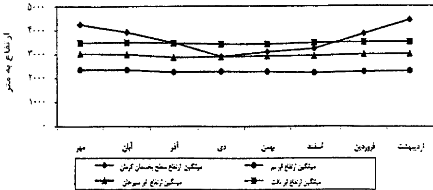
شکل ۷ نمودار مقایسه ارتفاع متوسط تراز یخبندان ایستگاه کرمان با ارتفاع ابر ایستگاه‌های بام، سیرجان و بافت
