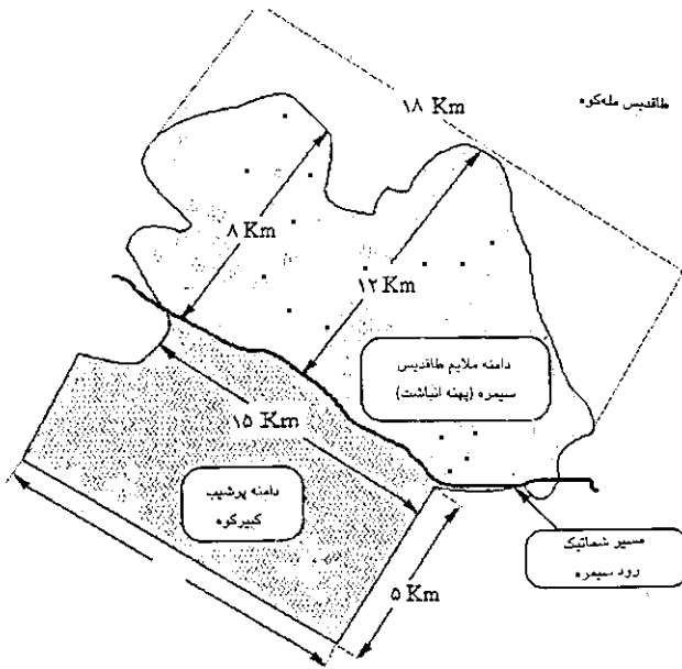
شکل ۳ طرح افقی لغزش در منطقه سیمره [۳]
