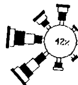
شکل ۴ گلباد سطح زمین ایستگاه کرمان در اسفند
