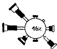
شکل ۲۱ گلباد سطح زمین ایستگاه بزد در بهمن
