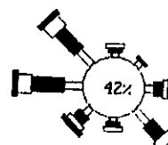
شکل ۲۲ گلباد سطح زمین ایستگاه بزد در اسفند
