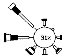
شکل ۲۵ گلباد سطح زمین ایستگاه شیراز در بهمن
