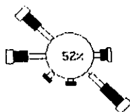
شکل ۲۰ گلباد سطح زمین ایستگاه بزد در دی
