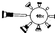
شکل ۱۷ گلباد سطح زمین ایستگاه اصفهان در بهمن
