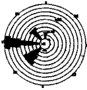
شکل ۴۶ - گلیاد تراز ۷۰۰ هکتوپاسکال ایستگاه بندرعباس در اسفند
