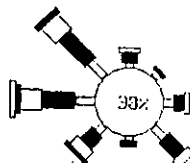
شکل ۲۳ گلباد سطح زمین ایستگاه بزد در فروردین
