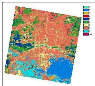
شکل ۵ نقشه طبقه‌بندی تصویر سال ۱۹۹۸
