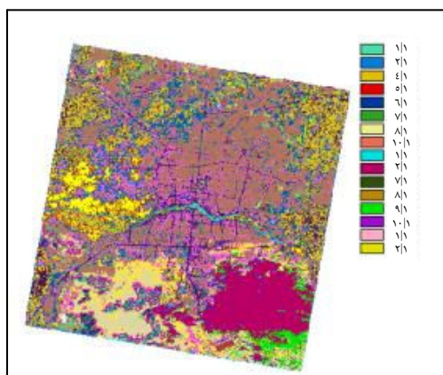
شکل ۶ نقشه حاصل از مقایسه طبقه‌بندیها
