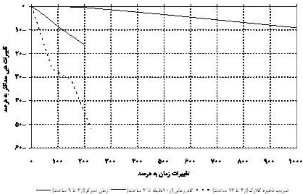
شکل ۱۱: بررسی تاثیرافزایش زمان تمرکز، گام زمانی و ضریب ذخیره کلارک بر دبی حداکثر سیلاب
