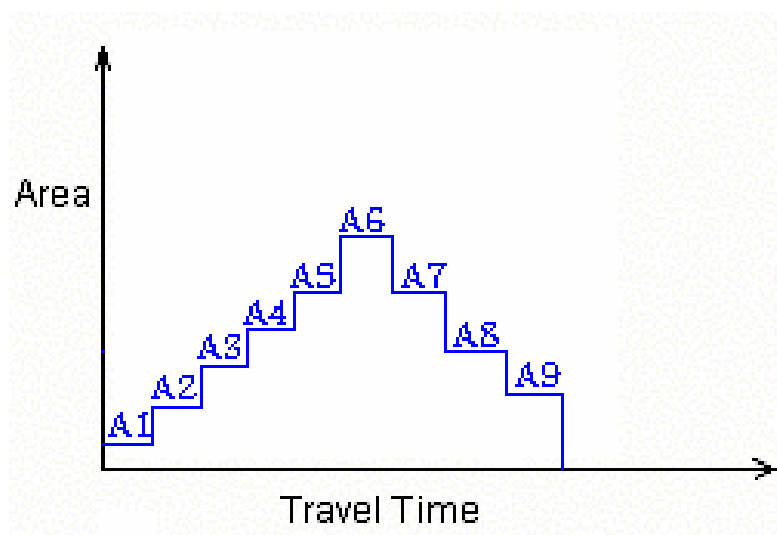
شکل ۲: هیستوگرام زمان - مساحت در یک حوضه فرضی
