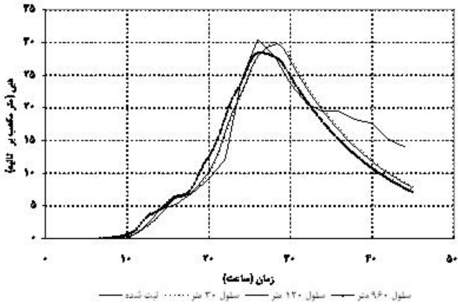
شکل ۱۲: مقایسه هیدروگراف های محاسبه شده با سلولهای ۹۶۰، ۱۲۰، و ۳۰ متر مربعی با هیدروگراف ثبت شده در تاریخ ۸۱/۱/۲۳
