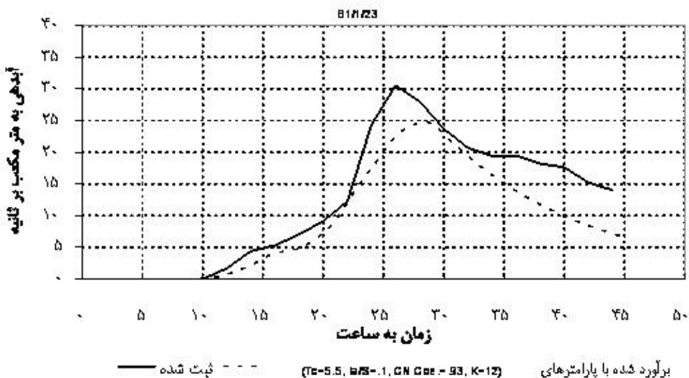
شکل ۱۰: اعتبار سنجی هیدروگراف سیلاب در ایستگاه آب سنجی سولقان در تاریخ ۸۱/۱/۲۳
