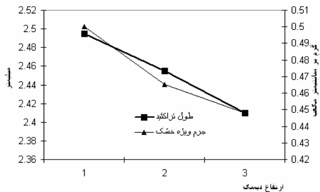
شکل ۱۱- تغییرات طول تراکتید و جرم ویژه خشک در محور طولی درخت
