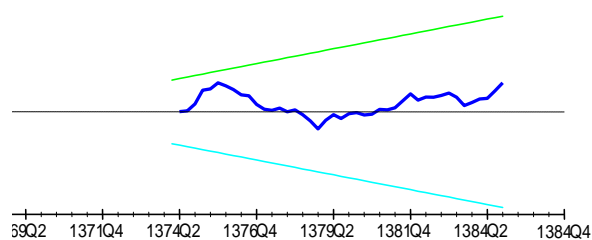
نمودار ۱- آزمون CUSUM تابع تقاضای پول ( M_1 )
