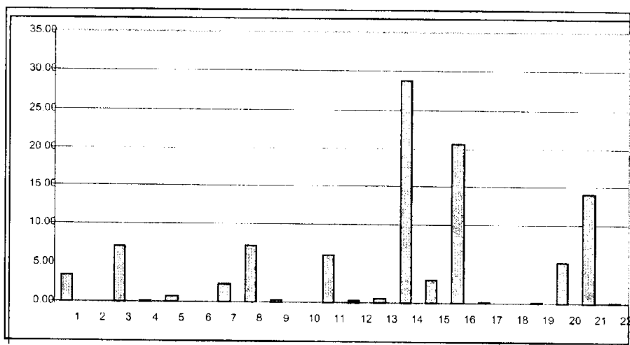
شکل ۱، نمودار درصد فراوانی ** حشرات انباری گنبد و مینودشت در طی سال‌های ۷۵-۷۶.
