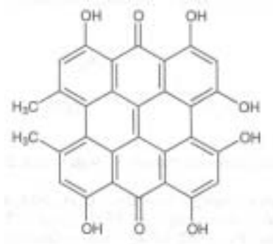
شکل شماره ۱- ساختمان شیمیایی هیپرسیسین
