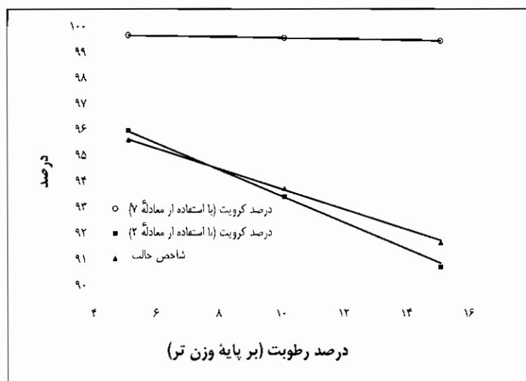
شکل ۵- نمودار تغییرات رطوبتی درصد کروییت و شاخص حالت دانه‌ها
