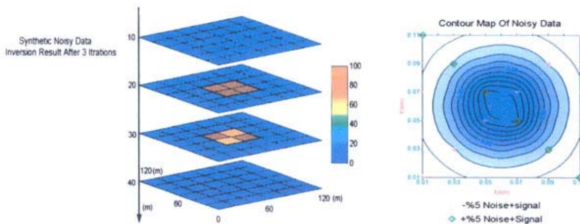
شکل 9 - الف) بی‌هنجاری ناشی از مدل مثال اول به همراه 5% نوفه روی قطر فرعی و 5% نوفه روی قطر اصلی بی‌هنجاری (سمت چپ)، ب) نتایج وارون سازی داده‌های نوفه‌ای نشان داده شده بعد از 3 تکرار با RMS = 1.21 \times 10^{-3} و همگرایی مطلوب مدل
