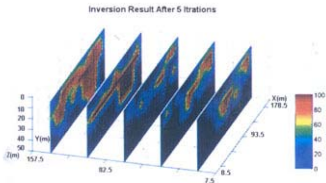
شکل 15: نتایج مدل‌سازی سه بعدی وارون و استفاده از درون‌یابی سه بعدی برای درک بهتر از بی‌هنجاری در 5 مقطع در راستای محور X با استفاده از داده‌های برداشت شده در معدن کرومیت
