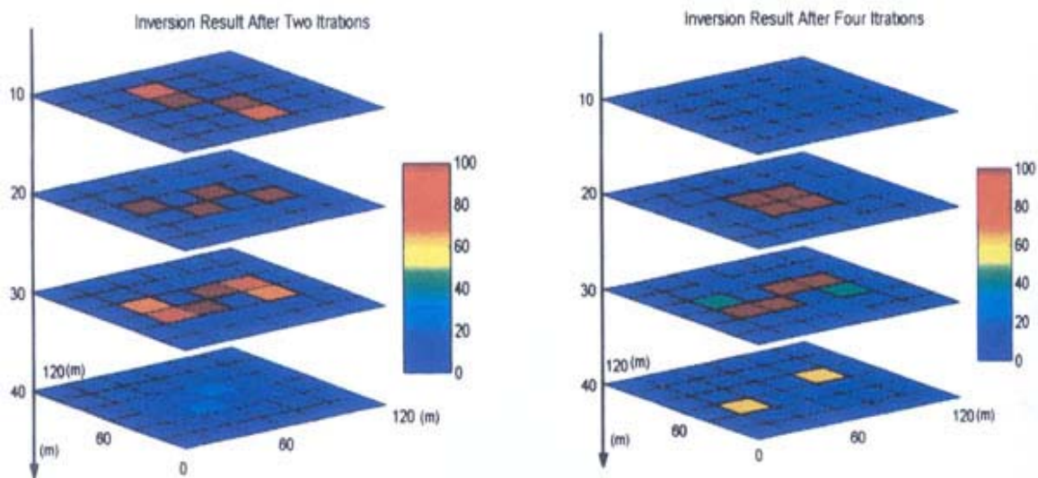
شکل 6 - الف) نتایج وارون سازی در تکرار دوم با RMS = 0.035 و توزیع کاملاً پراکنده چگالی‌ها در مدل (سمت چپ)، ب) نتایج وارون سازی در تکرار چهارم با RMS = 1.127 \times 10^{-6} و همگرایی نسبی مدل بعد از 4 تکرار
