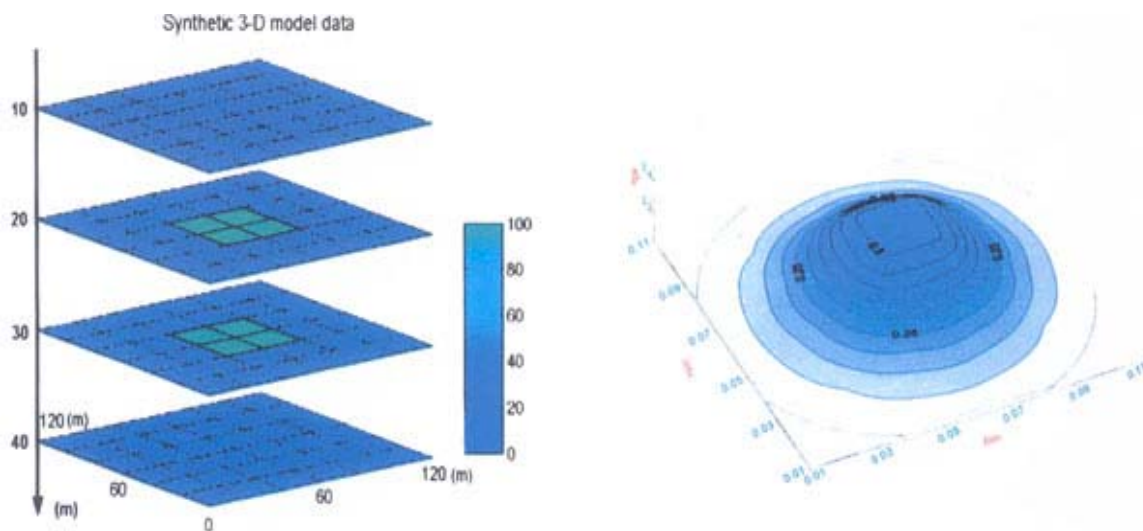
شکل 2 - الف- توزیع هندسی چگالیها در مدل مفروض (سمت چپ)، ب- بی‌هنجاری ناشی از مدل مفروض (سمت راست)
