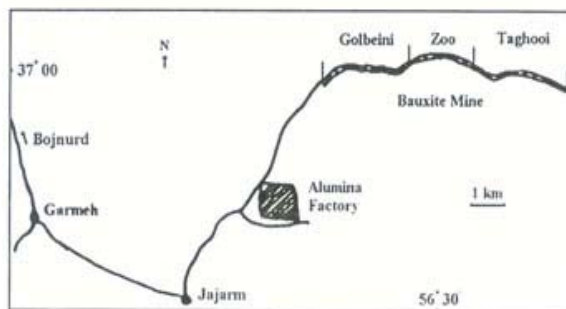
شکل ۱- موقعیت جغرافیایی و راههای دسترسی به برش مورد مطالعه.
