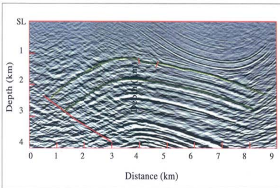
شکل 2- يك مقطع لرزه‌نگاري مهاجرت داده شده عمقي تفسیر شده در منطقه کرج و پارسی که برای انتخاب روش مناسب برای بازگرداندن، مورد استفاده قرار گرفته است.
