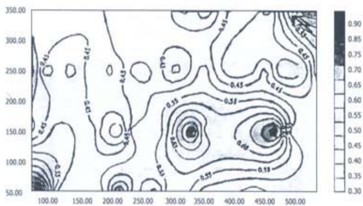
شکل 10- نقشه کنتوری اندیس سرستی شدگی ( K_2O/K_2O+Na_2O )
