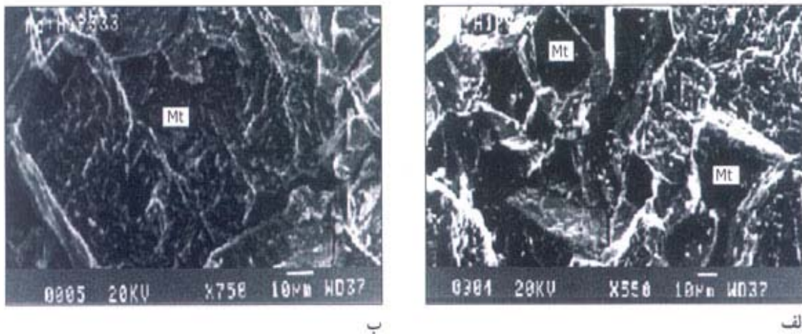
شکل 7- الف) یک تصویر SEM از بلورهای درشت مگنتیت با سطحی صاف و مرز مشخص با میانبرهای پیریتی بزرگنمایی 550 برابر ب) تصویر SEM با بزرگنمایی 750 برابر لایه‌بندی در بلورهای کانی فرو مغناطیس مگنتیت دیده می‌شود در گوشه سمت راست، بلور غیر مغناطیسی پیریت فاقد لایه‌بندی مشاهده می‌شود.
