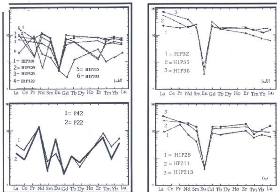
شکل 9- نمودار عنکبوتی تعدادی از نمونه‌های موجود در جدول 1 (الف) نمودار نمونه‌های برداشت شده از سنگ دیواره در پله شماره 3 (ب) نمودار نمونه‌های برداشت شده از آمفیبولهای همراه کانسار
