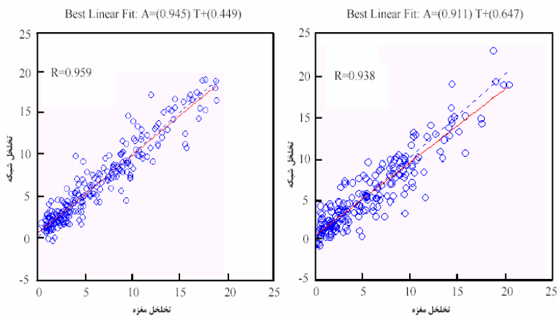
شکل ۶- نمودار مربوط به رابطه تخلخل مغزه و شبکه در مراحل آزمایش (شکل چپ) و تعمیم به چاه ۳۱ (شکل راست) برای شبکه با ۱۰ پارامتر ورودی
