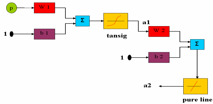
شکل ۴- طرح ساده‌ای از شبکه نفوذ پذیری مورد استفاده
