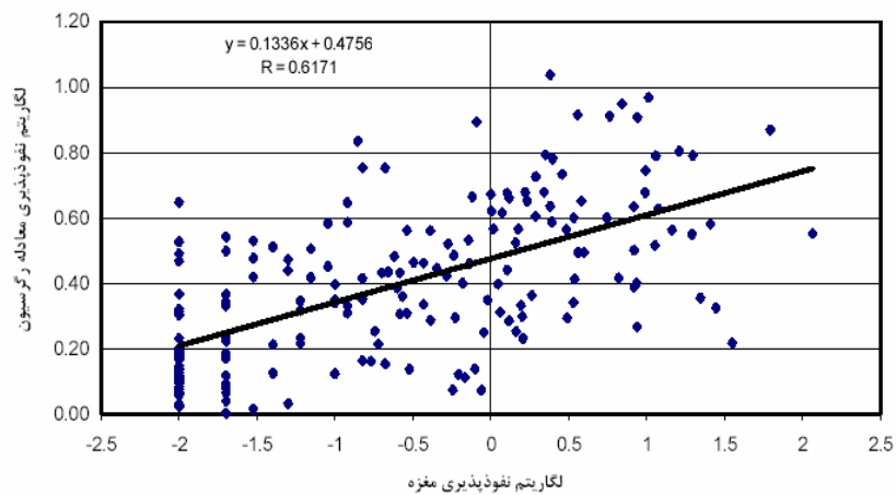
شکل ۱۰- نمودار مربوط به رابطه لگاریتم نفوذپذیری مغزه و معادله رگرسیون در چاه شماره ۳۱
