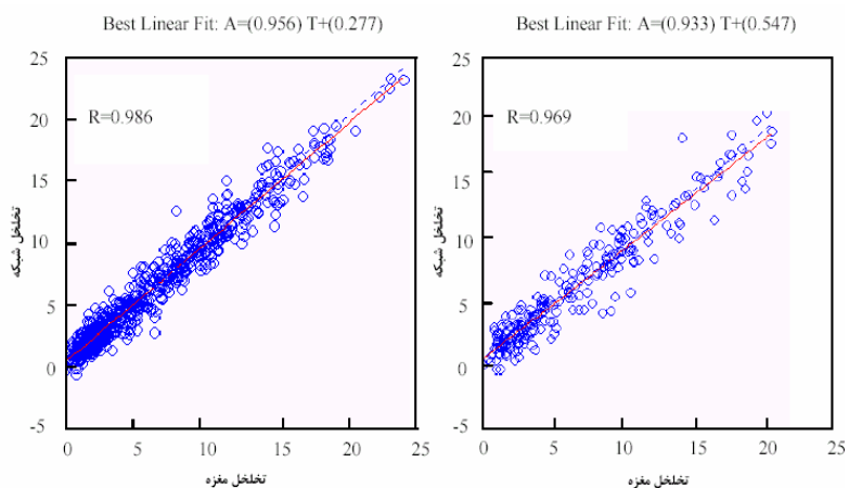
شکل ۵- نمودار مربوط به رابطه تخلخل مغزه و شبکه در مراحل آموزش (شکل چپ) و آزمون (شکل راست) برای شبکه با ۱۰ پارامتر ورودی
