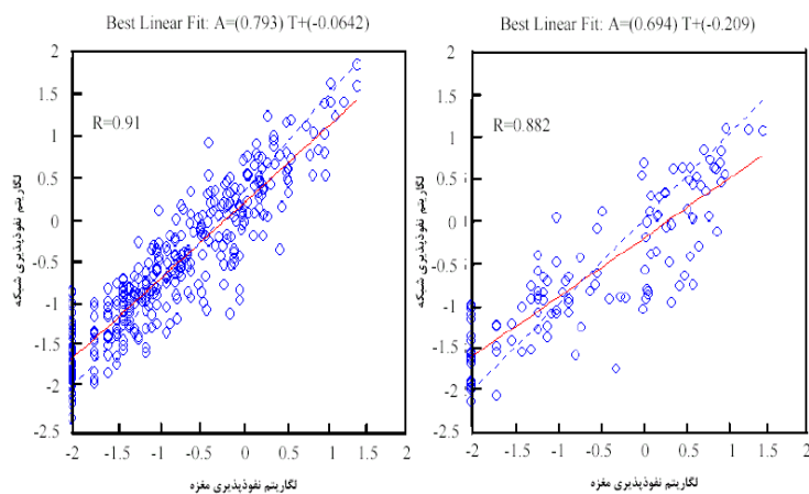
شکل ۷- نمودار مربوط به رابطه لگاریتم نفوذپذیری مغزه و شبکه در مراحل آموزش (شکل چپ) و آزمون (شکل راست) برای شبکه با ۱۱ پارامتر ورودی
