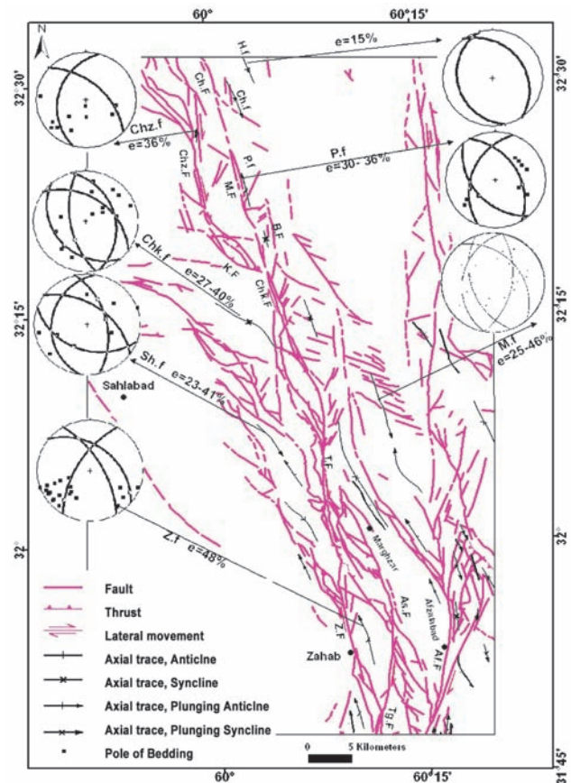
شکل ۷- تصاویر سیکلوگرافیک و تغییرات میزان کوتاه شدگی در چین های منطقه مورد مطالعه. علائم اختصاری: P.f چین پرنگ، H.f چین حسین آباد، Ch.f چین چاه خشکان، Chz.f چین چشمه زنگی، Chk.f چین چاخو، Sh.f چین شورک، Z.f چین زهاب، M.f چین مرغزار
