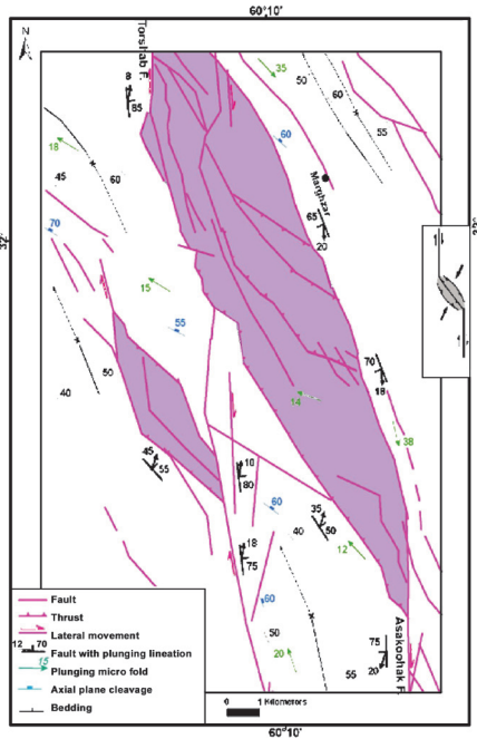
شکل ۶- نقشه ساختاری منطقه فشاری آساکوهاک
