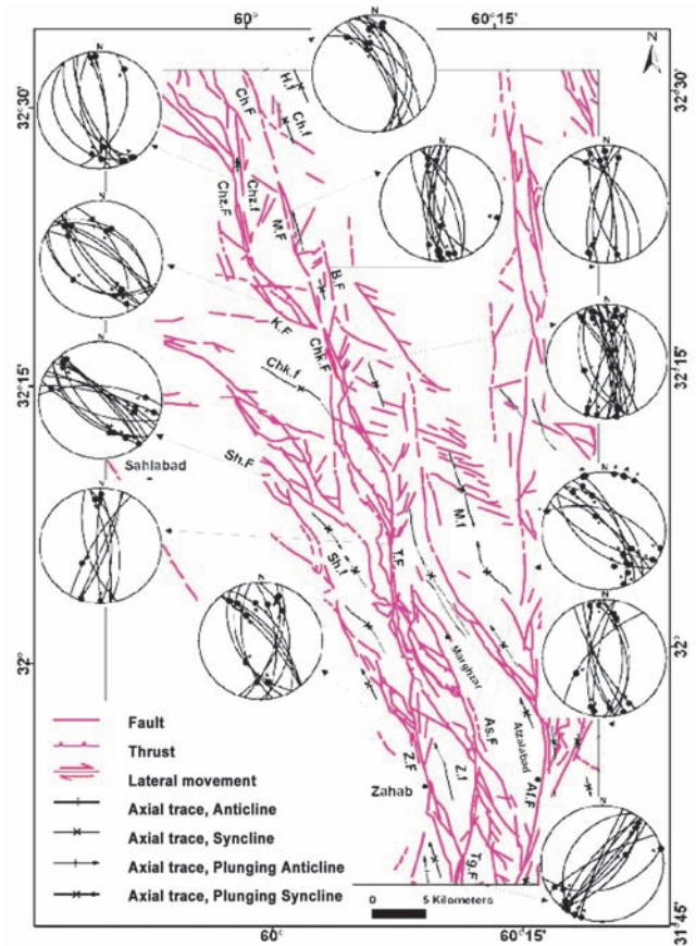
شکل ۲- نقشه گسل‌ها با نمایش تصاویر سیکلوگرافیک و چین‌ها در منطقه مطالعه. علائم اختصاری: گسل چاه خشکان، Ch.F، گسل چشمه‌زنگی، B.F، گسل بهارمز، M.F، گسل معروفان، Chk.F، گسل چاخو، K.F، گسل کسراب، T.F، گسل ترشاب، Sh.F، گسل شورک، As.F، گسل آساکوهک، Z.F، گسل زهاب، A.F، گسل افضل آباد، Tg.F، گسل تگ سیاه. علائم اختصاری مربوط به چین‌ها: H.f، چین حسین آباد، Ch.f، چین چاه خشکان، Chz.f، چین چشمه زنگی، Chk.f، چین چاخو، Sh.f، چین شورک، Z.f، چین زهاب، M.f، چین مرغزار
