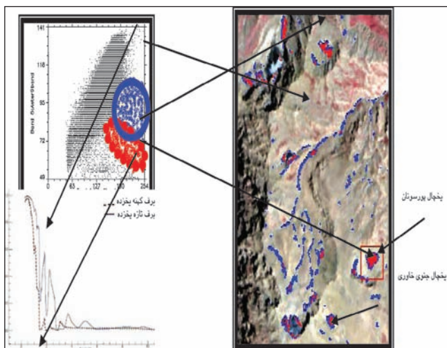
شکل ۸- مناطق مختلف برفی بر روی تصویر Aster و فضای عارضه مربوط به باندهای ۵ و ۹
