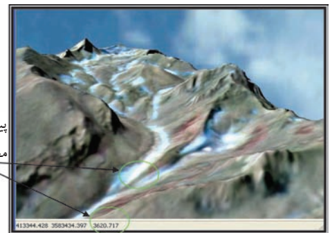
شکل ۱۱- مدل ارتفاعی منطقه یخچالی و تصویر تلفیق شده Aster و IRS
