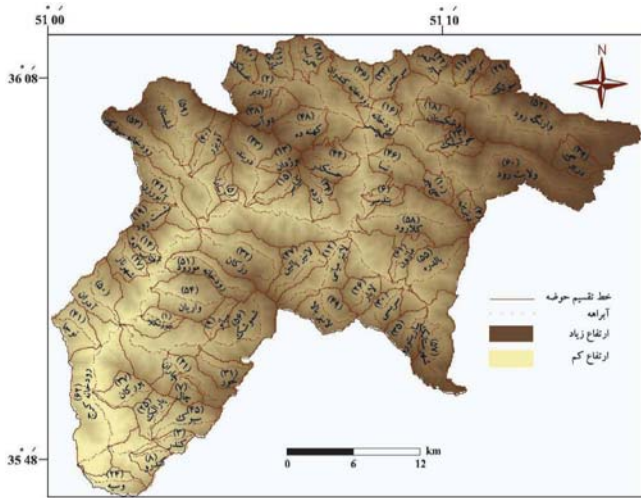
شکل ۳- زیر حوضه‌ها و آبراهه‌های به دست آمده از مدل ارتفاعی-رقومی حوضه زهکشی کرج.
