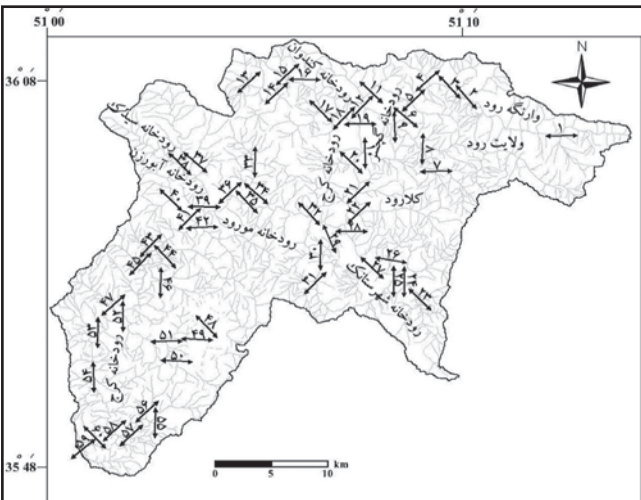
شکل ۵- محل مقاطع اندازه‌گیری شاخص نسبت عرض کف دره به ارتفاع آن (Vf)، در حوضه کرج.
