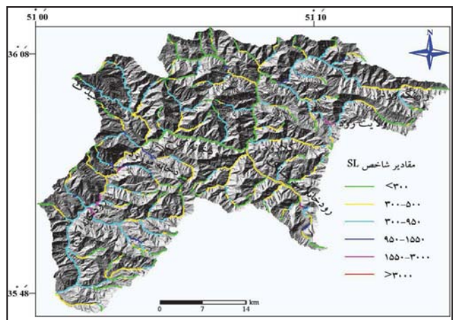
شکل ۴- توزیع میزان شاخص طول-شیب آبراهه‌ها (SL)، در شبکه زهکشی رودخانه کرج.
