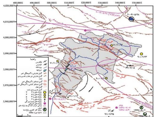
شکل ۲- نقشه لرزه‌زمین‌ساخت ناحیه مورد مطالعه. مختصات ناحیه بر اساس سیستم UTM است (Nazari, 2005).
