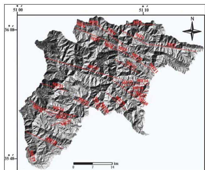
شکل ۶- خطوط مستقیم به عنوان پیشانی‌های گسلی منطقه برای محاسبه مقادیر شاخص پیشانی کوه (Smf).
