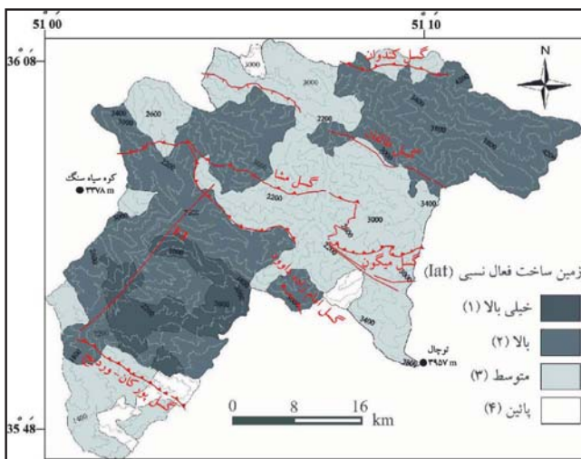
شکل ۷- پراگندگی شاخص زمین‌ساخت فعال نسبی (Iat) در حوضه رودخانه کرج و ارتباط آن با گسل‌های ناحیه.
