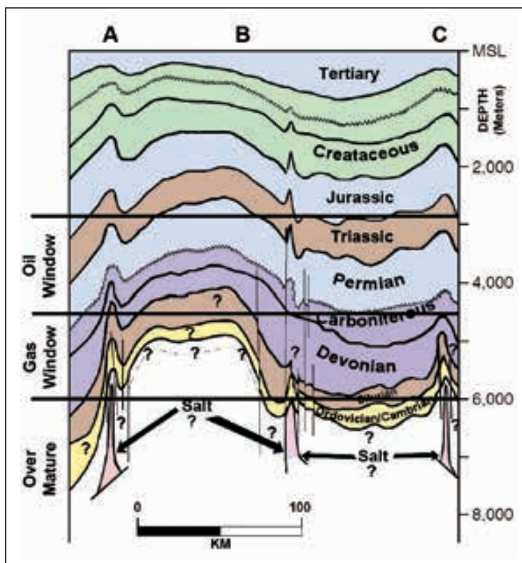
شکل ۸- طرح نمادین از روند ABC (باختری- خاوری) در شکل ۳ که از چاه A، چاه B (کمان قطر) و چاه C عبور می‌کند. در این شکل چاه B بر روی یک بلندای قدیمی (میدان پارس جنوبی) و با ویژگی‌های کم ستبرایی از رسوبات رویی آن دارای ساختار تله‌ای بسیار مناسبی برای به دام انداختن هیدروکربورهای زایش یافته از مناطق اطراف خود است.
